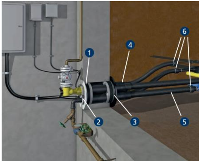
Bild 3: Mauerdurchführung mit Hilfe einer Mehrspartenhauseinführung
